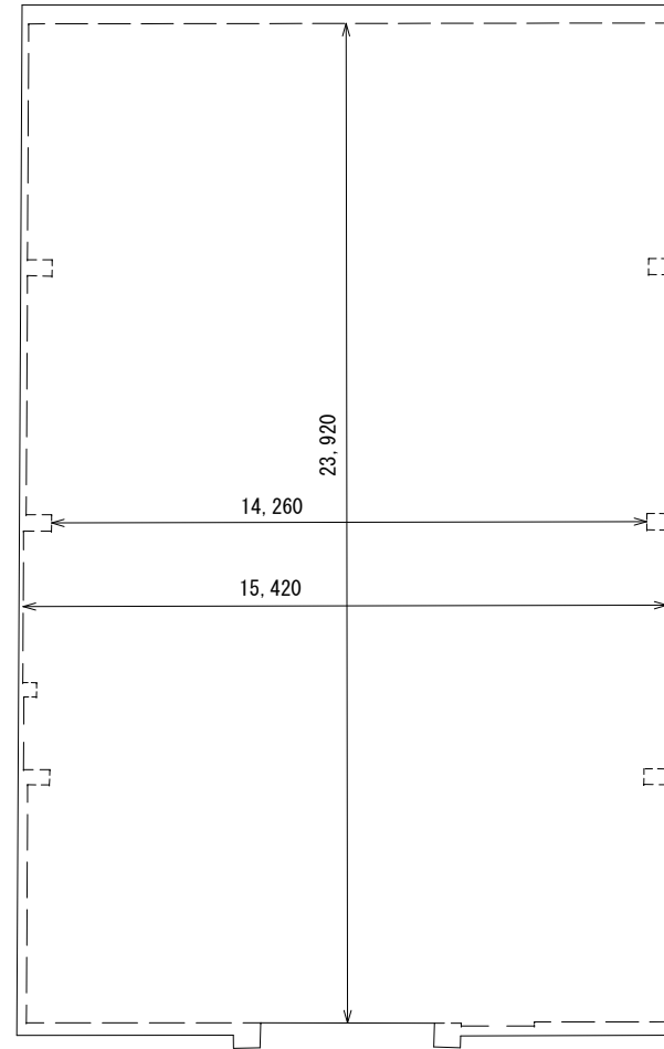
平面図
