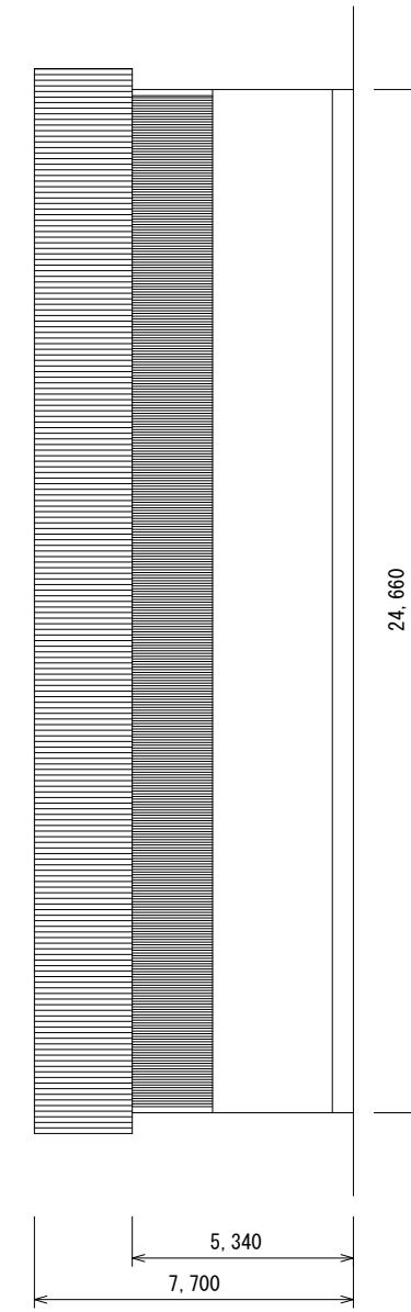
東側立面図
