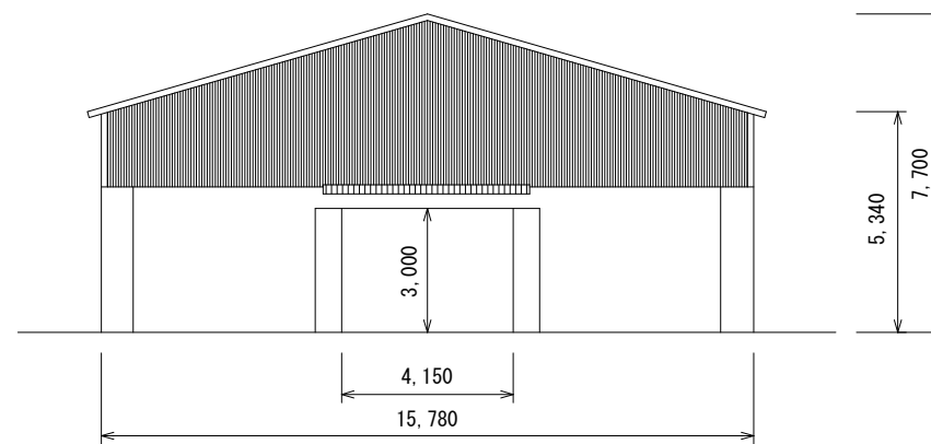
南側立面図
