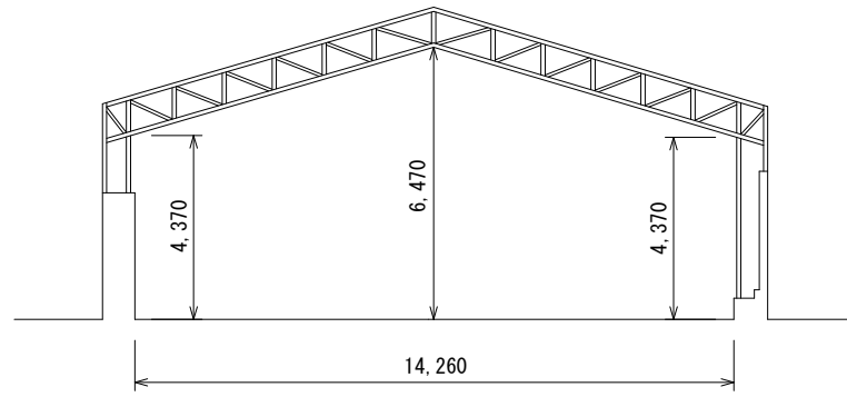
室内断面図
