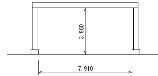
室内断面図
