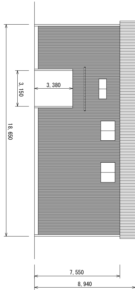
西側立面図
